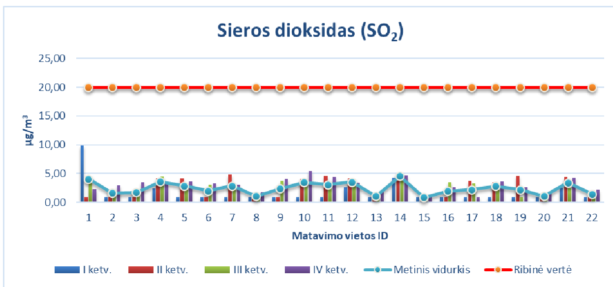
11 pav. \text{SO}_2 koncentracijų pasiskirstymai Kėdainių rajone
