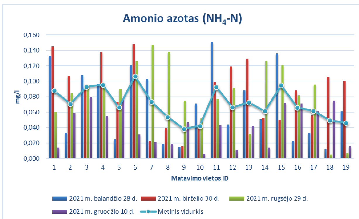
21 pav. Amonio azoto koncentracijos kitimas per 2021 m. (Ribinė vertė >2 \text{ mgN/l} , Ribinė vertė grafike neatvaizduojama nes gautos koncentracijos ženkliai mažesnės už ribinę vertę.)
