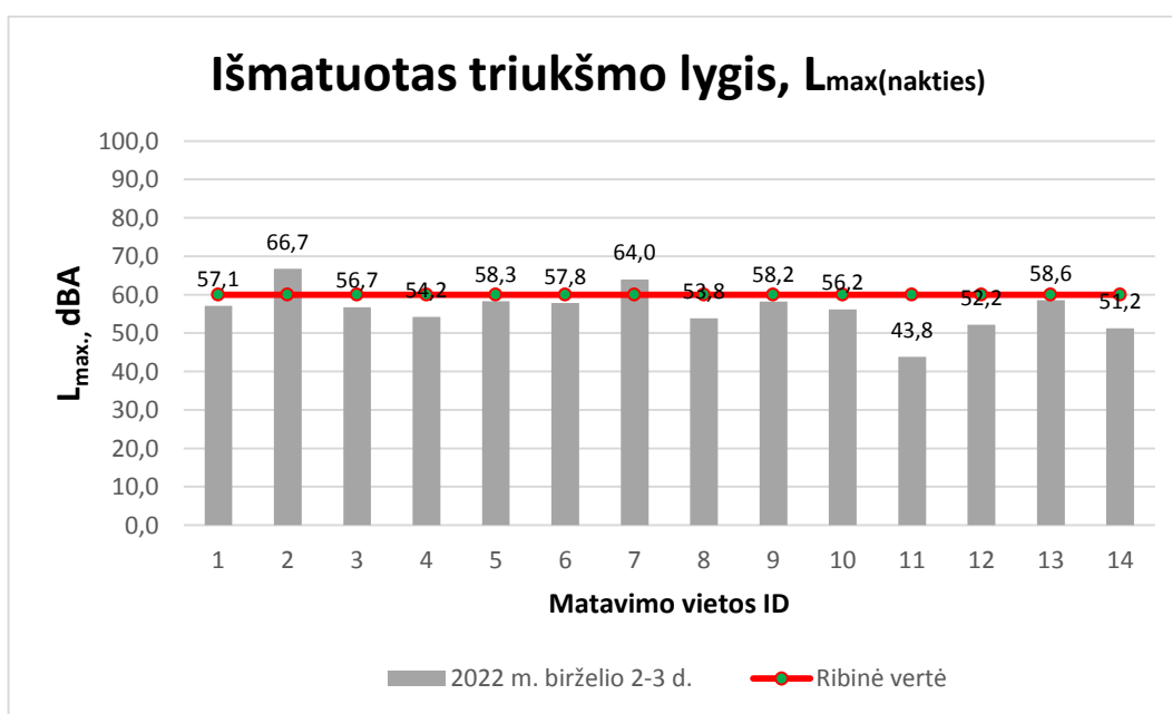
62 pav. Maksimalaus triukšmo pasiskirstymas matavimo vietose nakties metu (22-7 val.).
