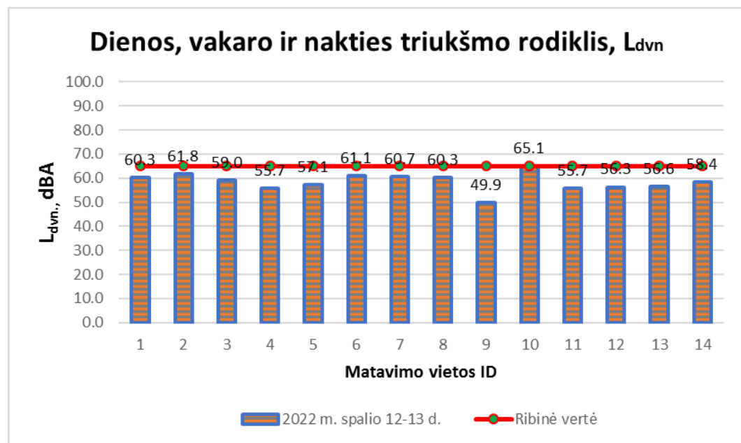
80 pav. Dienos, vakaro ir nakties triukšmo rodiklio ( L_{dvn} ) pasiskirstymas matavimo vietose.
