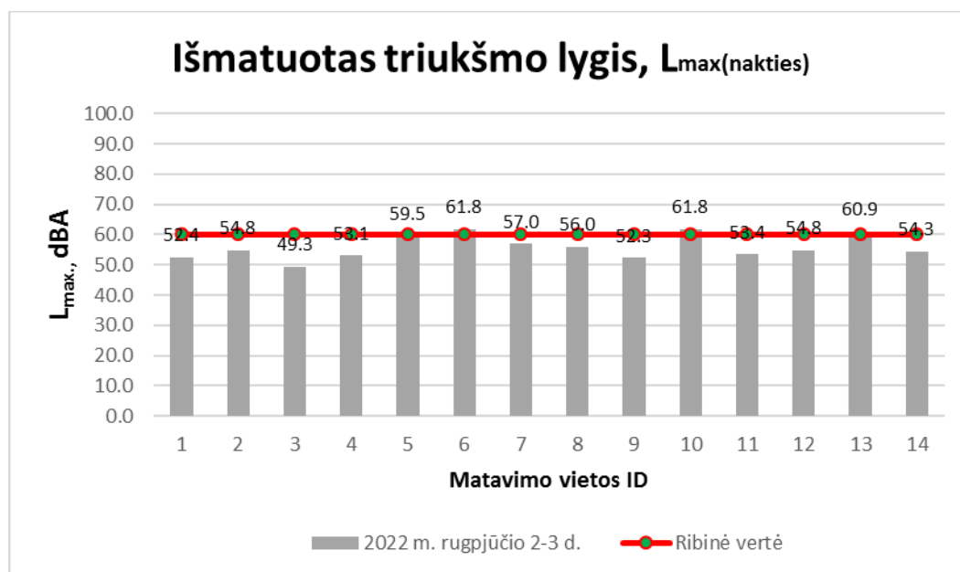
70 pav. Maksimalaus triukšmo pasiskirstymas matavimo vietose nakties metu (22-7 val.).
