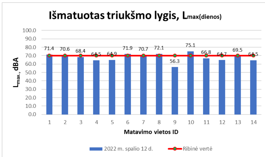
74 pav. Maksimalaus triukšmo pasiskirstymas matavimo vietose dienos metu (7-19val.). Ribinis dydis 70 dBA.
