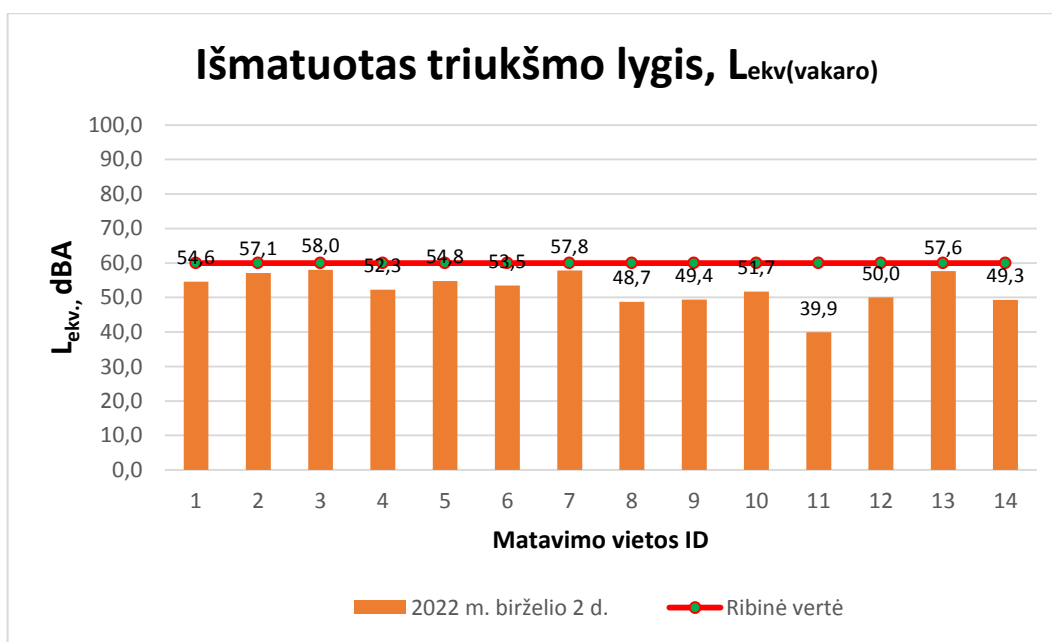
69 pav. Ekvivalentinio triukšmo pasiskirstymas matavimo vietose vakaro metu (19-22 val.).
