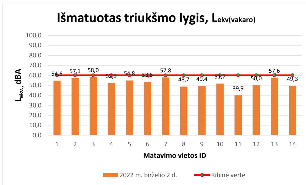
61 pav. Ekvivalentinio triukšmo pasiskirstymas matavimo vietose vakaro metu (19-22 val.).
