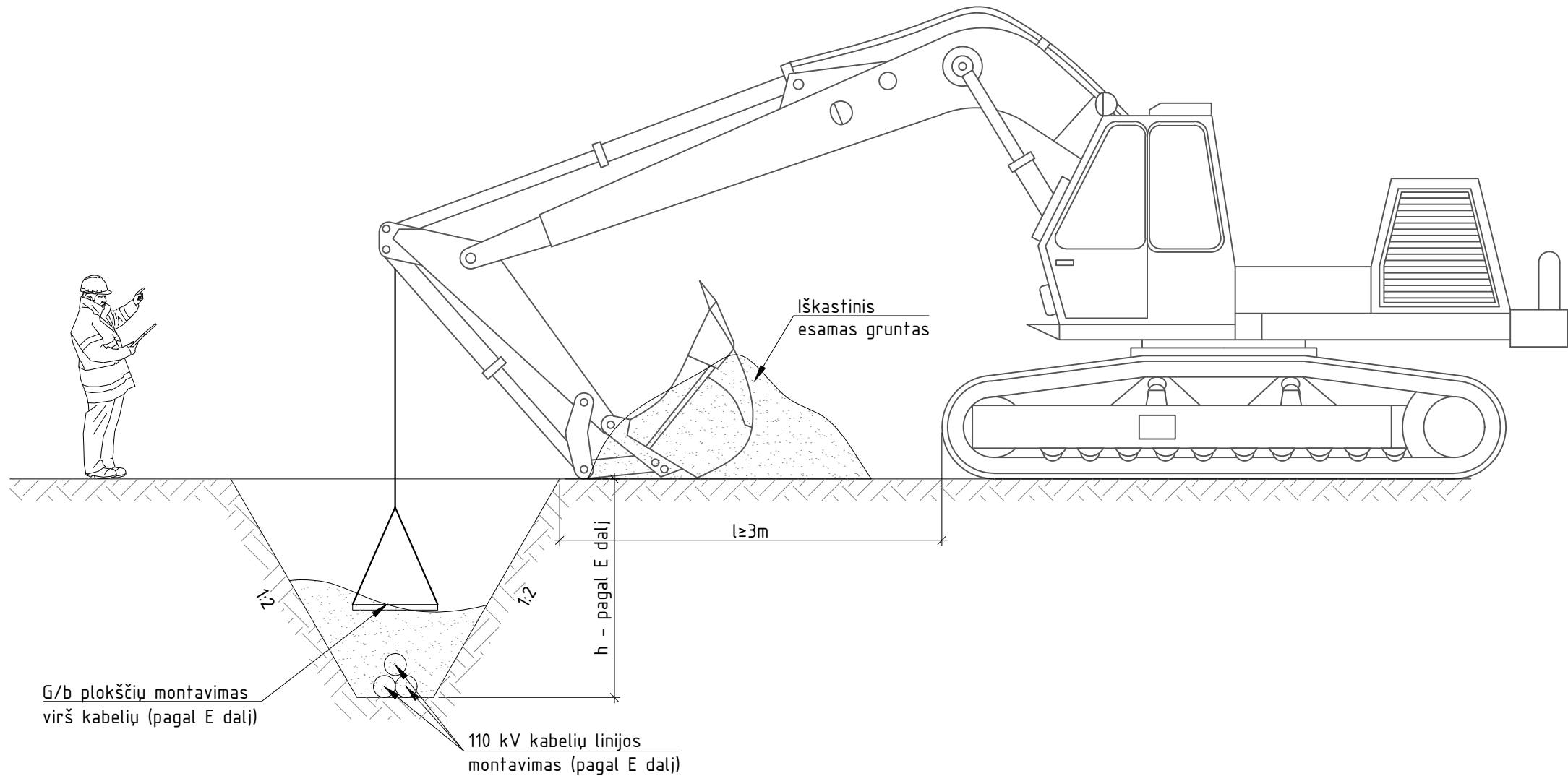
Kabelinių linijų tranšėjose principinė montavimo schema
