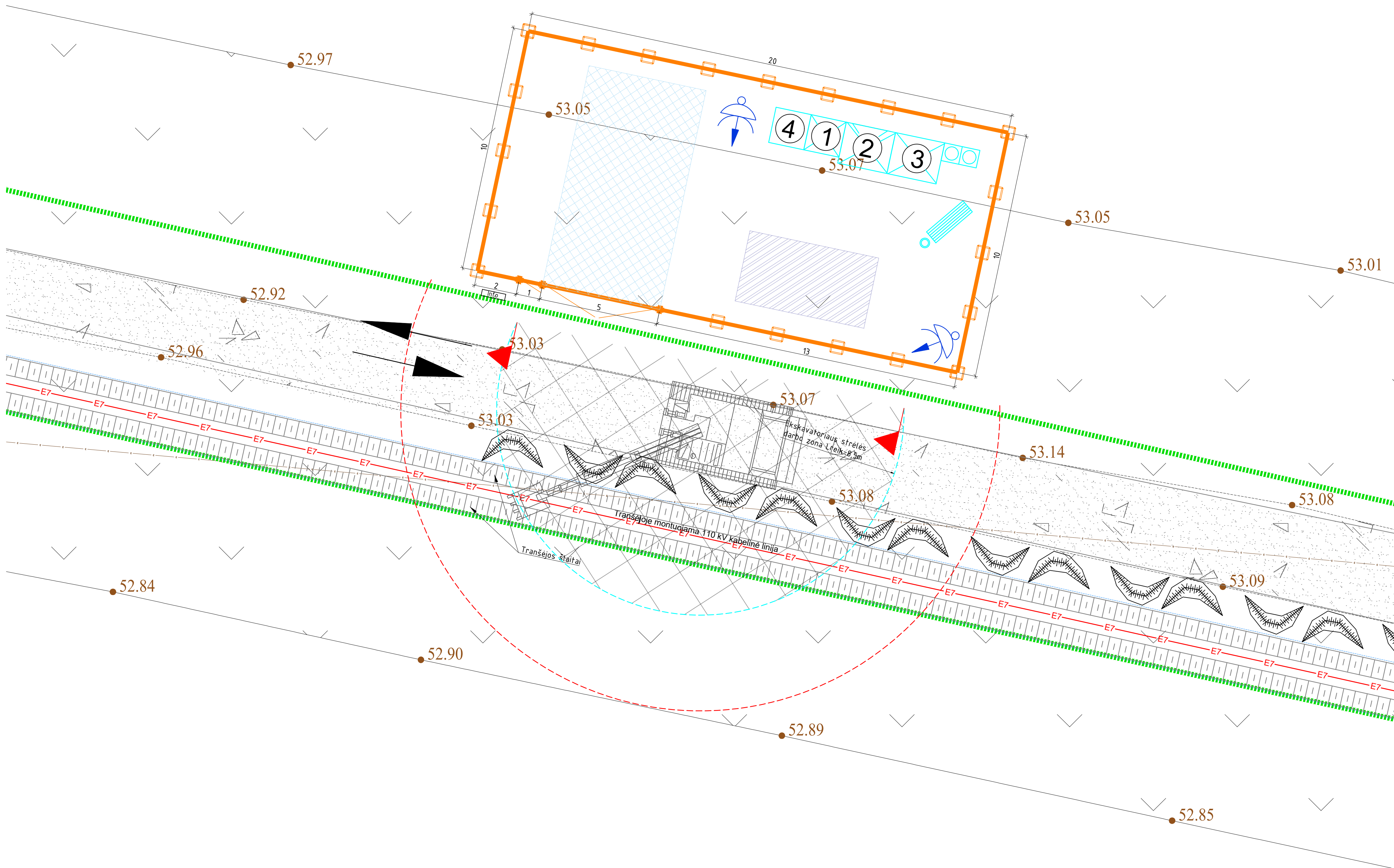
Kabelinių linijų tranšėjose principinė montavimo schema
