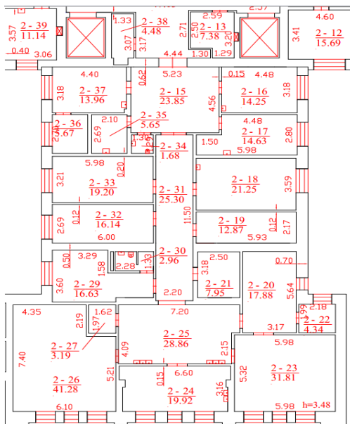
Esama patalpų schema
