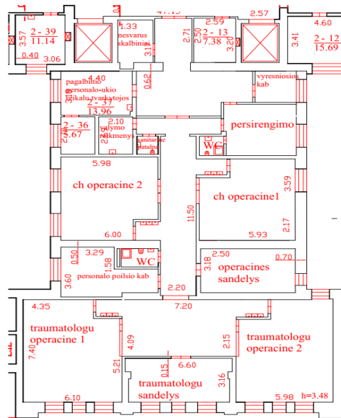
Patalpų schema po remonto
