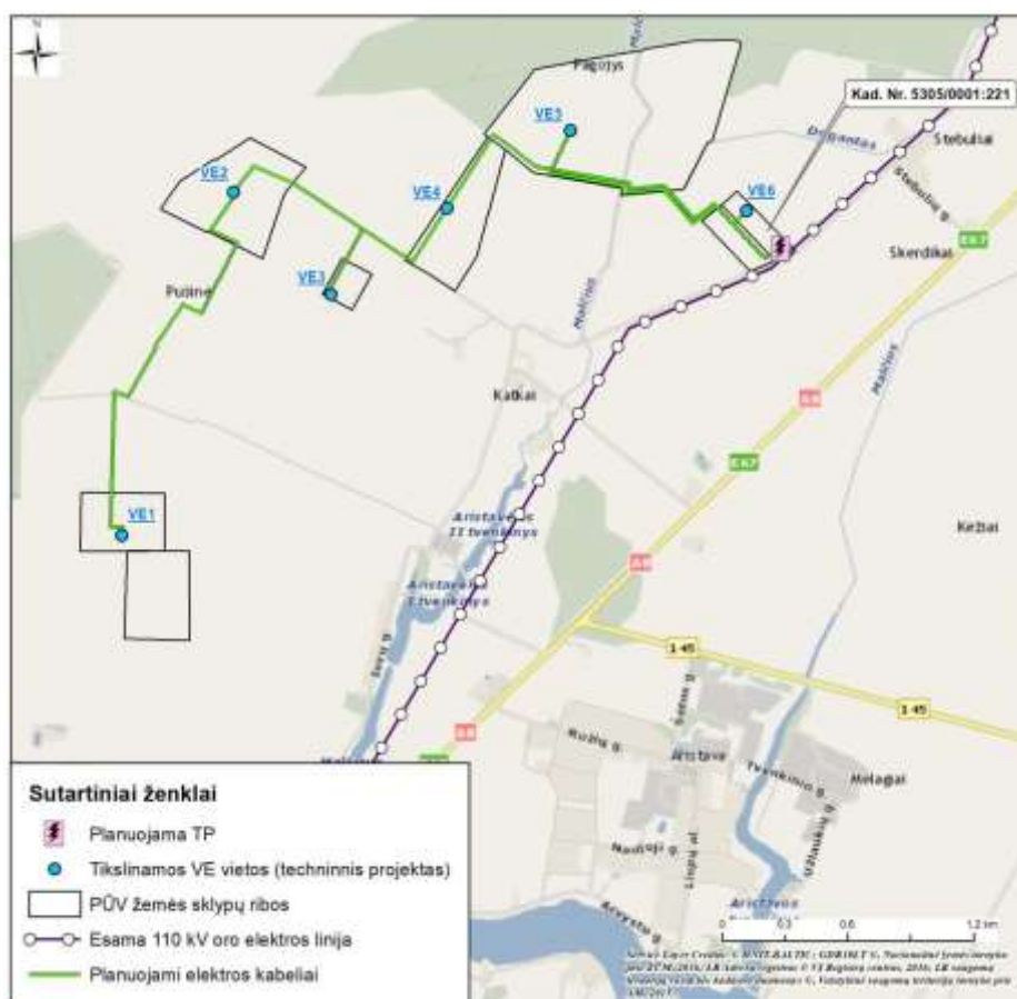
2.2 pav. Planuojamos transformatorinės pastotės vieta.
