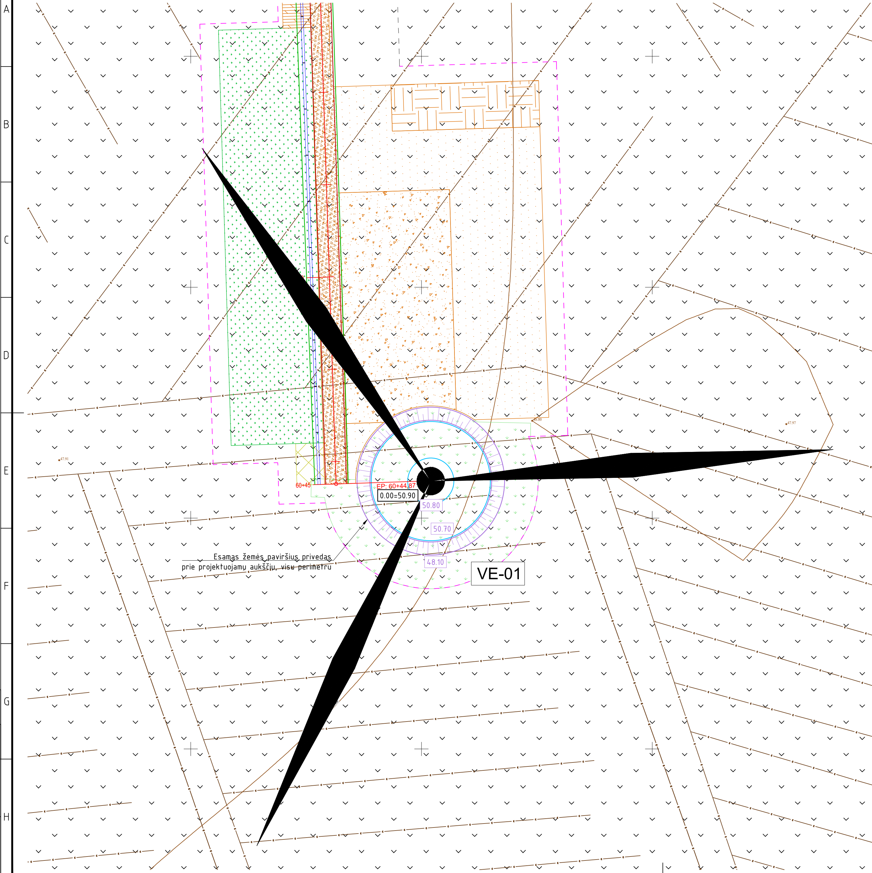
Sklypo aukščių planas M1:500
