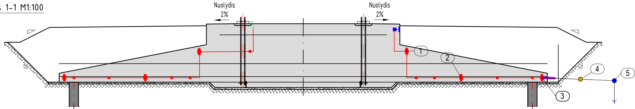
Pjūvis 1-1 M1:100
