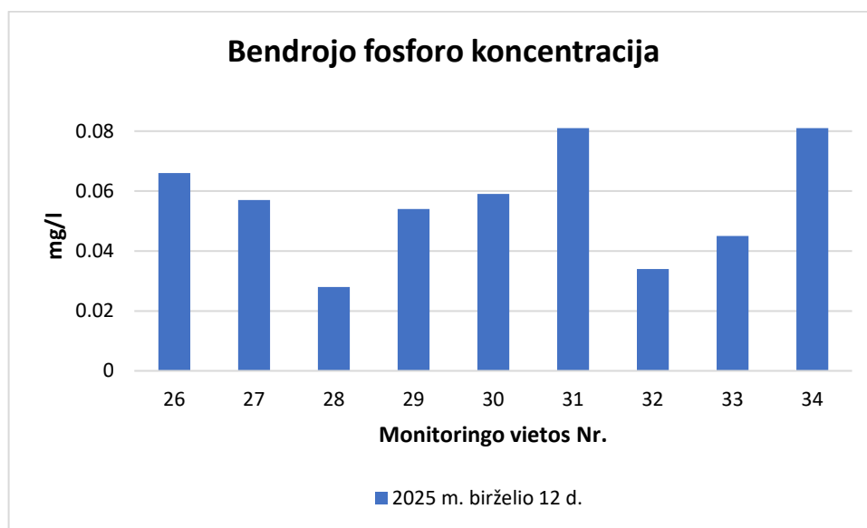
32 pav. Bendrojo fosforo koncentracijų pasiskirstymas Kėdainių rajono savivaldybės drenažo sistemų nuvedamo vandens monitoringo vietose 2025 m. II ketv. (Ribinė vertė 4 mg/l grafike neatvaizduojama, nes gautos koncentracijos ženkliai mažesnės už ribinę vertę)
