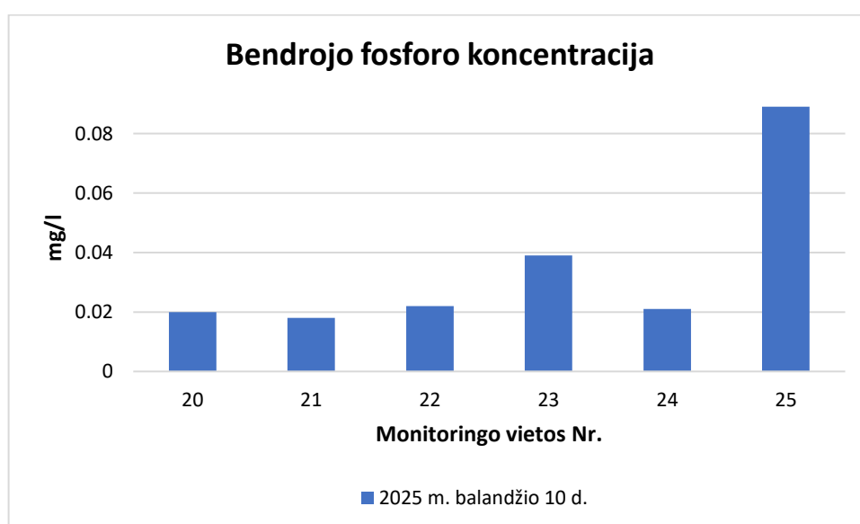
29 pav. Bendrojo fosforo koncentracijų pasiskirstymas Kėdainių rajono savivaldybės paviršinio tvenkinių vandens monitoringo vietose 2025 m. II ketv. (Ribinė vertė 1,6 mg/l grafike neatvaizduojama, nes gautos koncentracijos ženkliai mažesnės už ribinę vertę)
