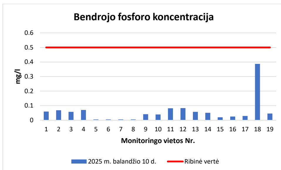
25 pav. Bendrojo fosforo koncentracijų pasiskirstymas Kėdainių rajono savivaldybės paviršinio upių vandens monitoringo vietose 2025 m. II ketv.
