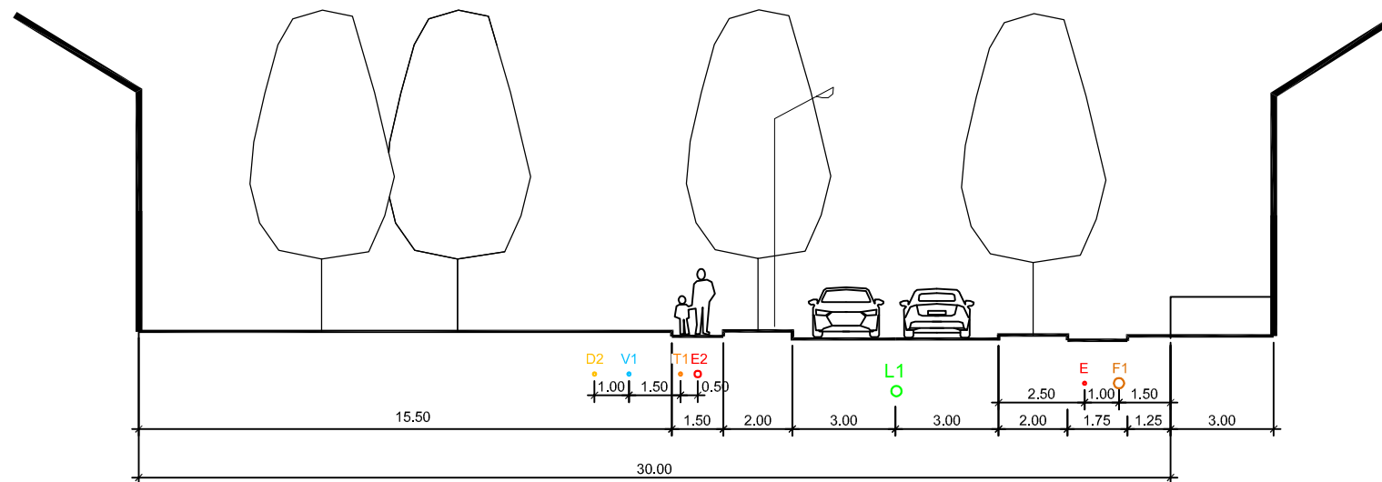
GATVĖS PJŪVIS 1-1, M 1:500
