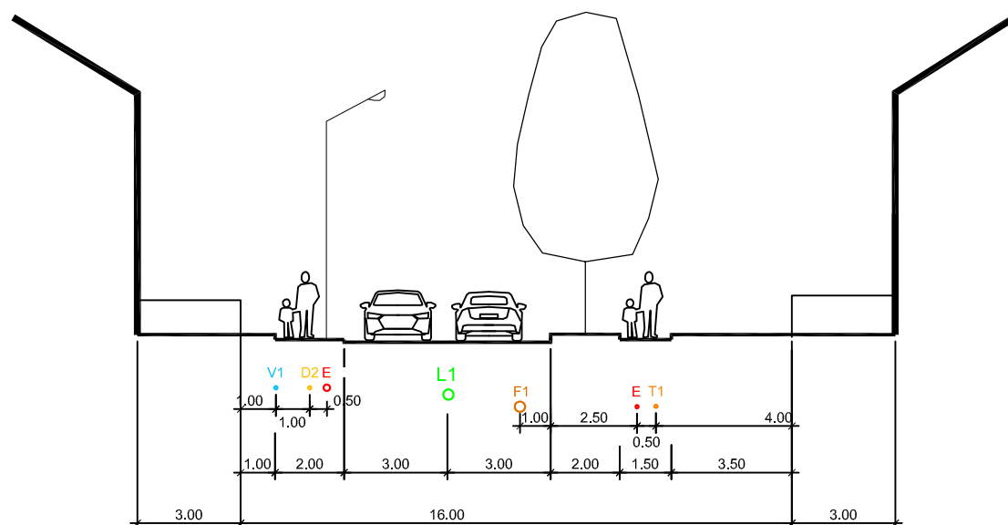
GATVĖS PJŪVIS 2-2, M 1:500
