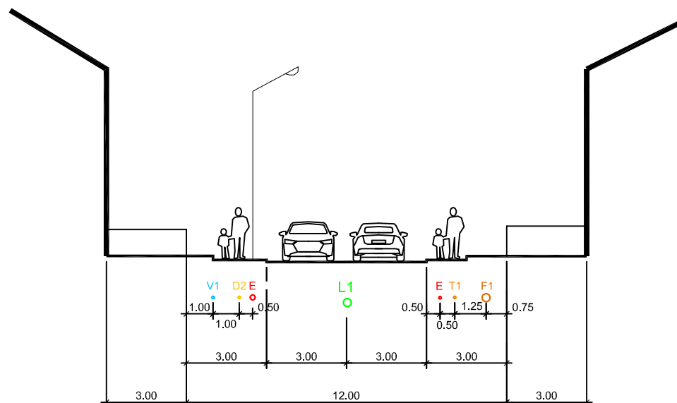
GATVĖS PJŪVIS 3-3, M 1:500
