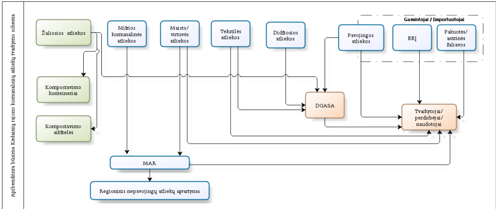
Priedas 4 Apibendrinta būsima komunalinių atliekų tvarkymo schema
